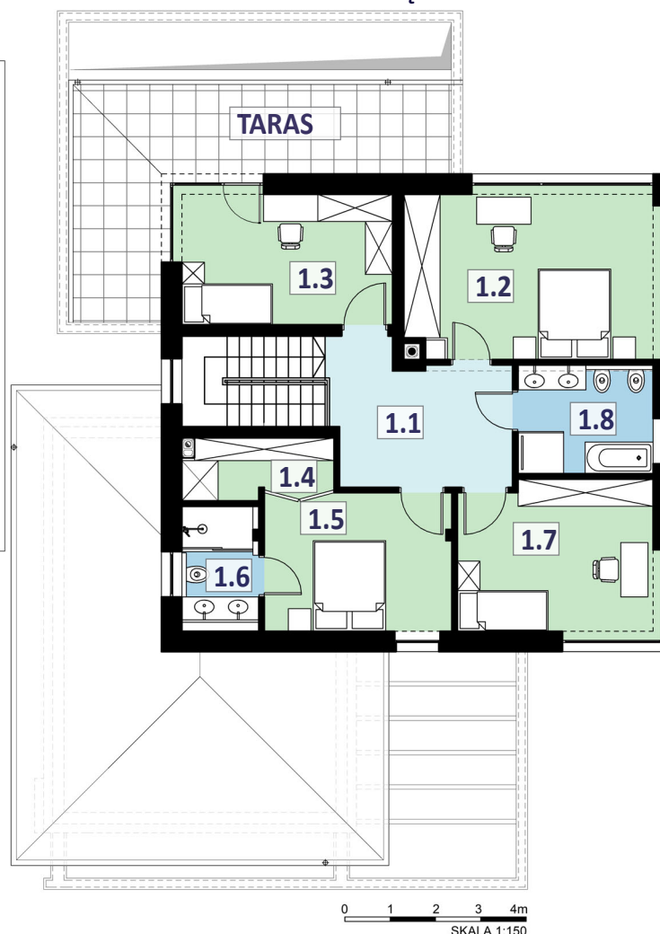
RZUT 1 PIĘTRA
