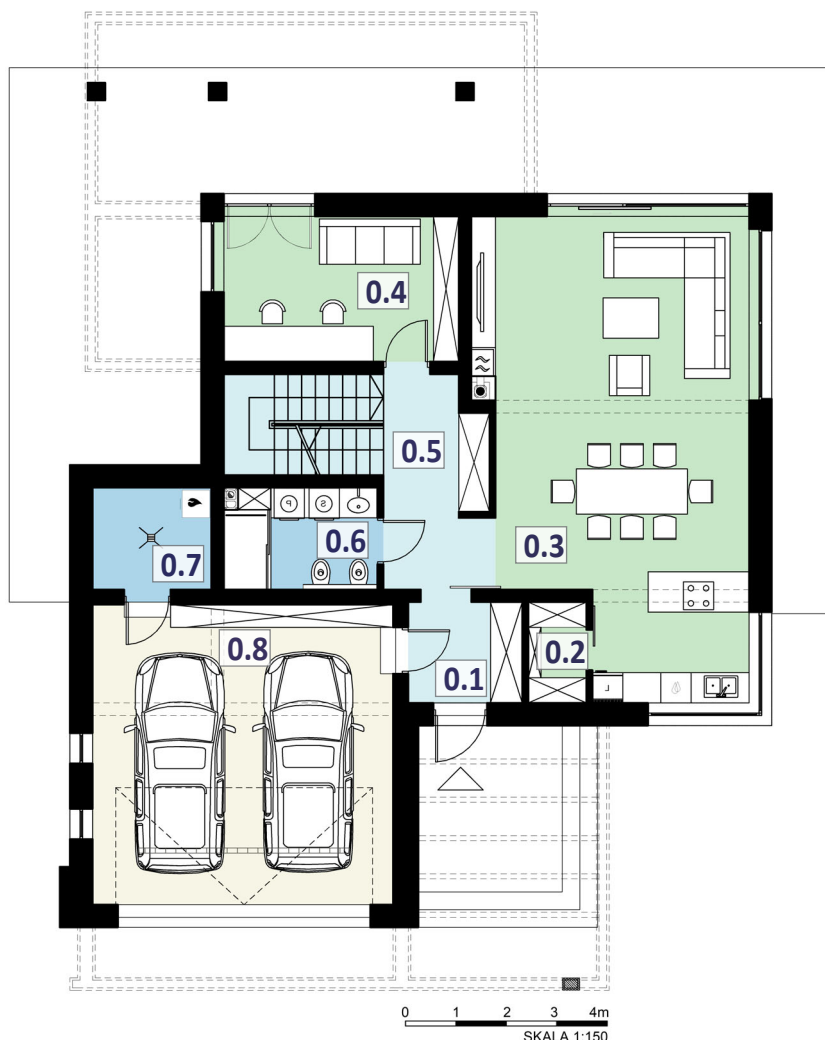
RZUT PARTERU
