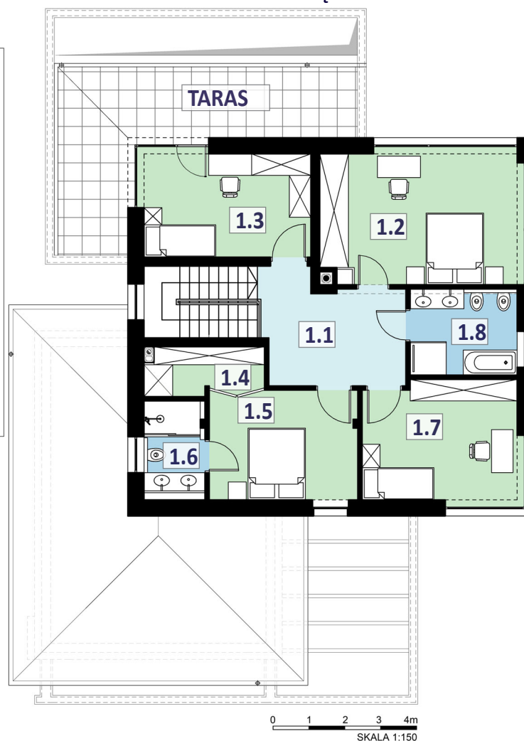
RZUT 1 PIĘTRA
