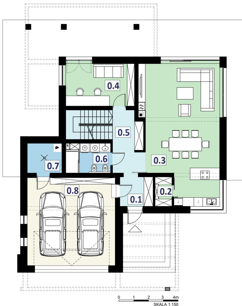
RZUT PARTERU
